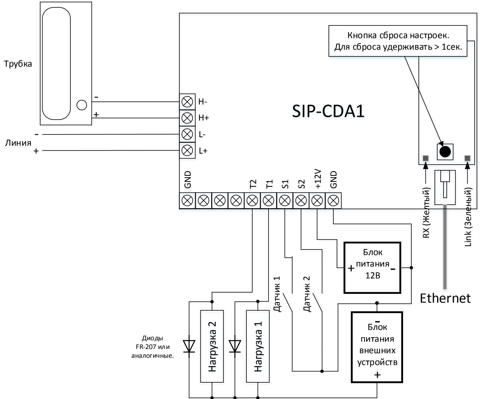
Схема подключения SIP-CDA1.
