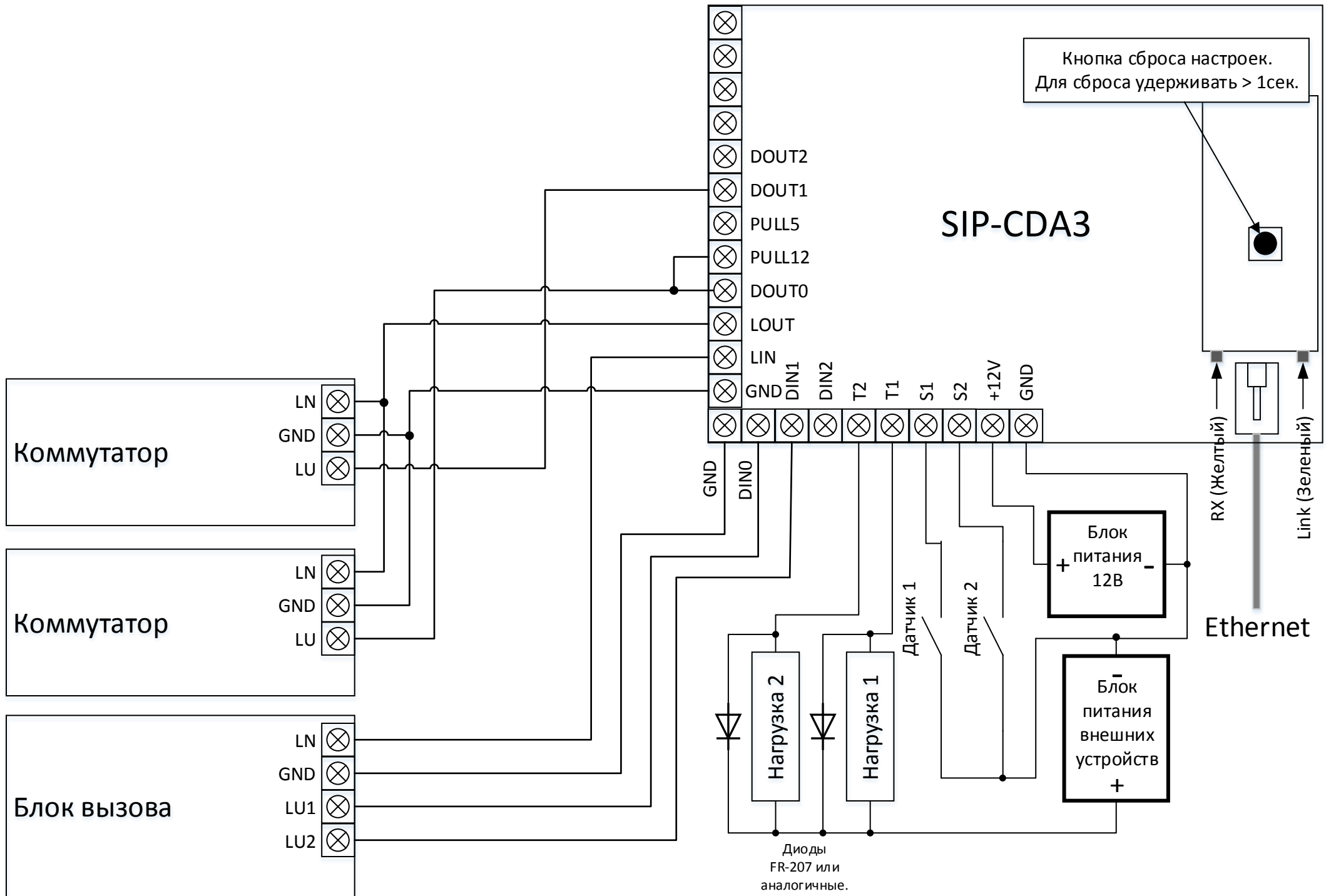
Схема подключения SIP-CDA3 к домофонам Цифрал.
